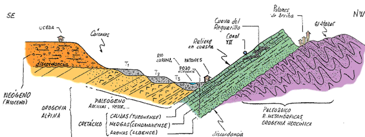
Perfil geológico Uceda-Patones de Arriba, en el entorno del azud de Valdentes
