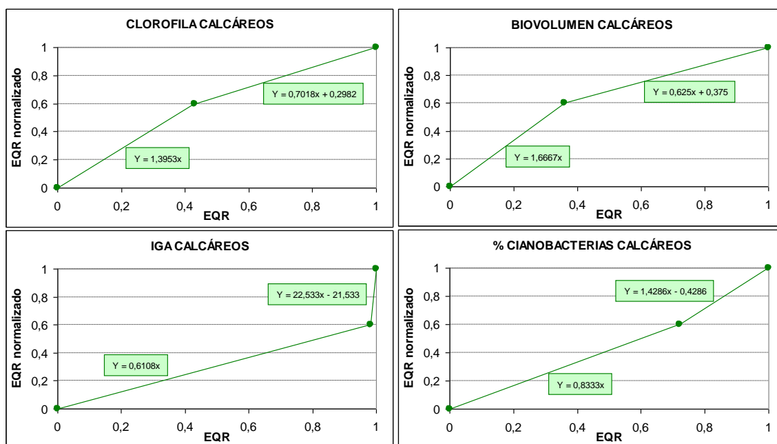
Figura 22. Gráficos con ecuaciones de normalización de EQR para tipologías 7, 8, 9, 10, 11 y 12.
