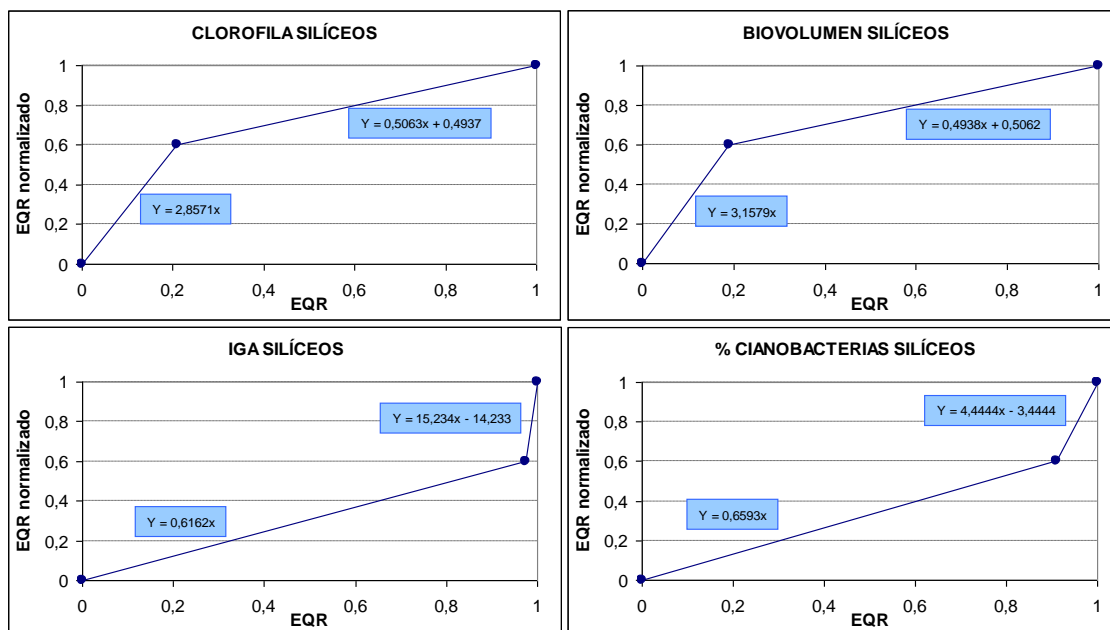
Figura 21. Gráficos con ecuaciones de normalización de EQR para tipologías 1, 3, 4, 5 y 6
