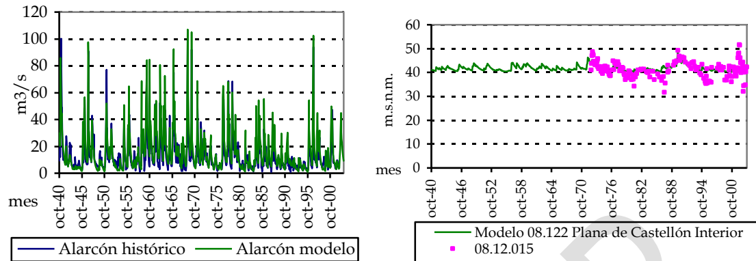
Figura 6. Caudales mensuales en régimen natural al embalse de Alarcón ( m^3/s ), y niveles piezométricos en la Plana de Castellón (m.s.n.m.). Contraste entre el modelo y los datos históricos.
