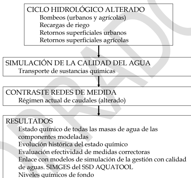
Figura 2. Metodología para la simulación de la calidad del agua, resultados y aplicaciones.
