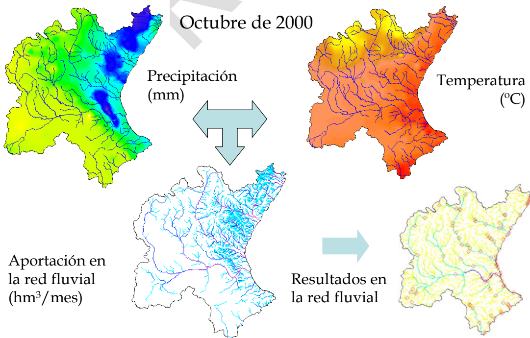
Figura 5. Precipitación temperatura y aportación en la red fluvial en octubre de 2000.
